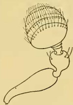
FIG. 3.— Cryphalus squamulosus Strohmeyer. Antenna. 12 × vergrössert.
